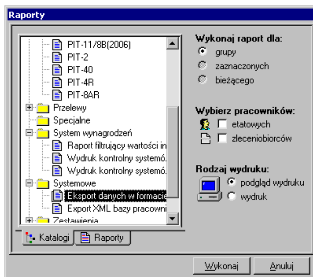
Rys. 3-11 Okno Raporty.
