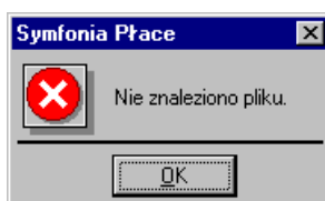
Rys. 4-23 Przykładowy komunikat.
