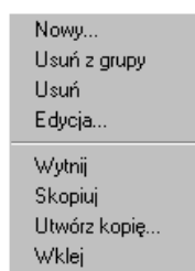
Rys. 4-25 Menu podręczne.
